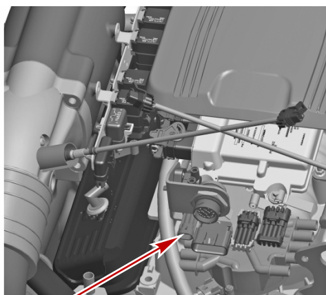
Connexion du faisceau d'alimentation – 5.0 MPI ECT
