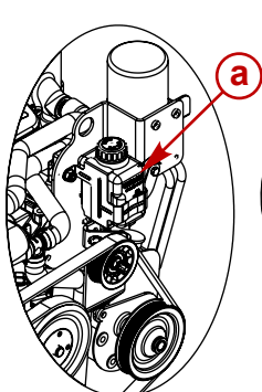
Contrôleur de graissage d'embases des moteurs 4.3 EC, modèles à refroidissement par eau de mer
