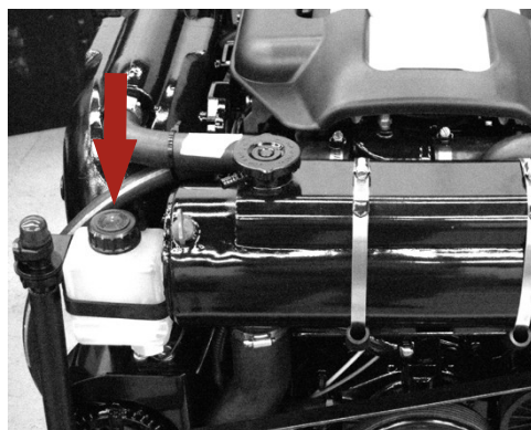
Contrôleur de graissage d'embase des moteurs 4.3 EC, modèles à refroidissement fermé
