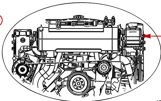
Contrôleur de graissage d'embases des moteurs 4.3 EC, modèles à refroidissement par eau de mer
