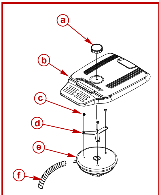
Capot moteur 5.0 EC
